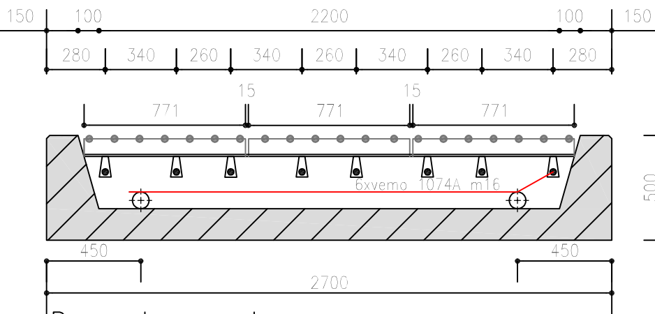
Dwarsdoorsnede
