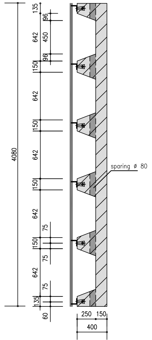
Langsdoorsnede
