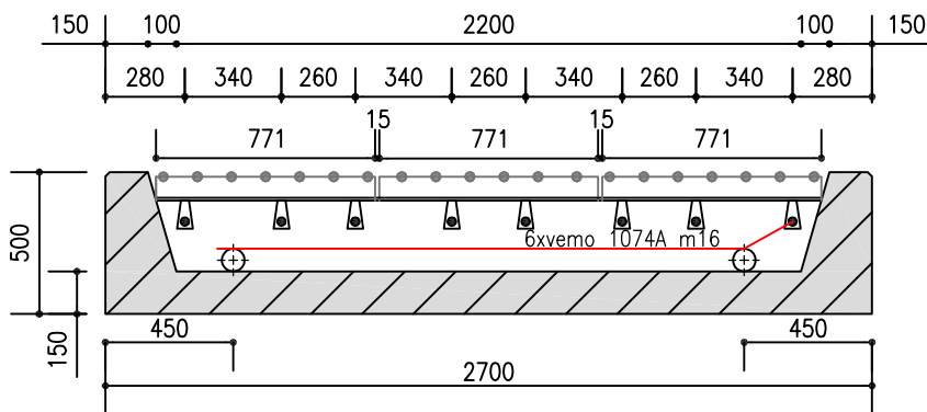
Dwarsdoorsnede
