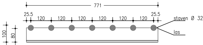
Aanzicht L 80.80.10
