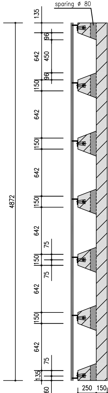
Langsdoorsnede
