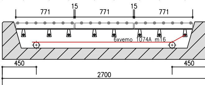
Dwarsdoorsnede
