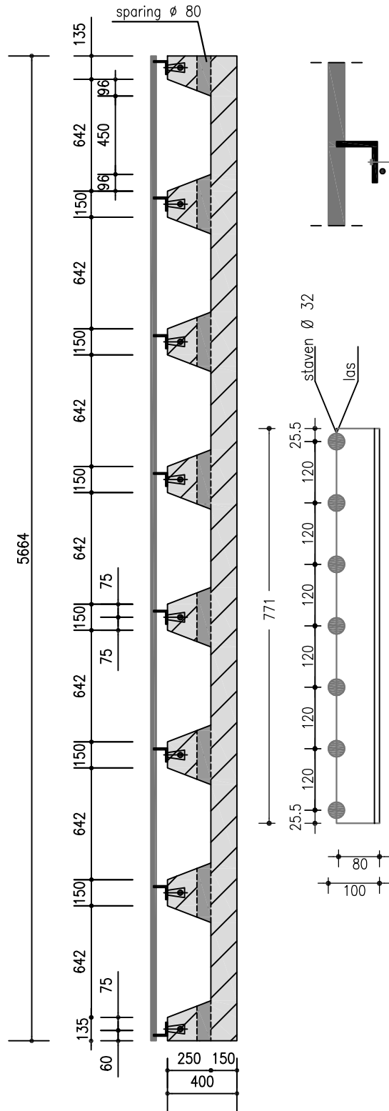
Langsdoorsnede
