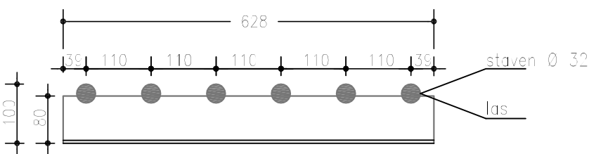
Aanzicht L 80.80.10
