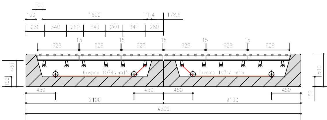
Dwarsdoorsnede
