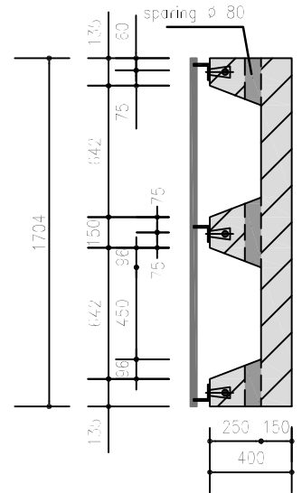
Langsdoorsnede
