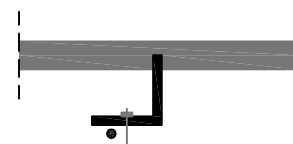
Doorsnede L 80.80.10
