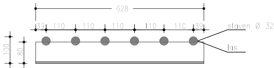
Aanzicht L 80.80.10
