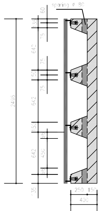
Langsdoorsnede
