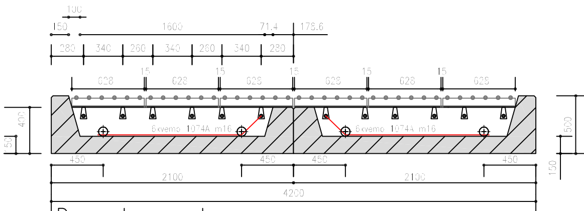
Dwarsdoorsnede
