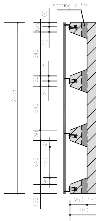
Langsdoorsnede
