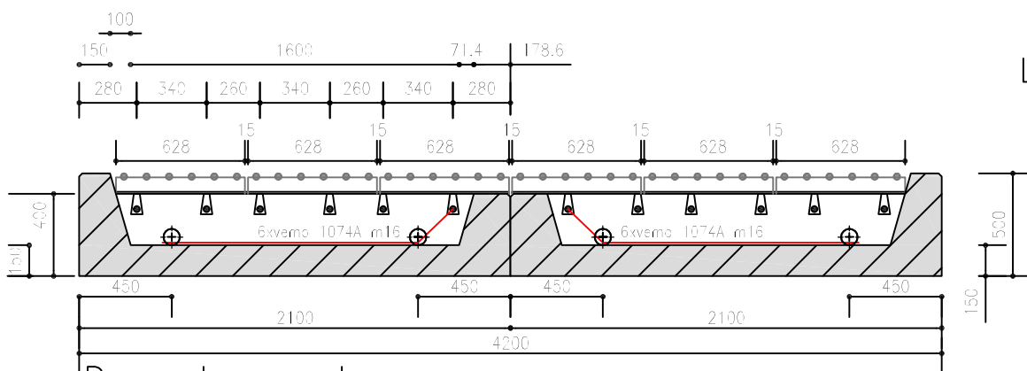
Dwarsdoorsnede
