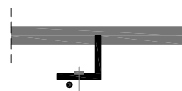
Doorsnede L 80.80.10
