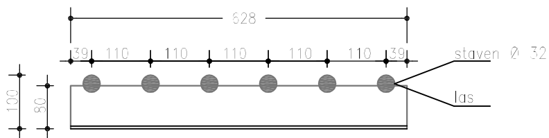
Aanzicht L 80.80.10
