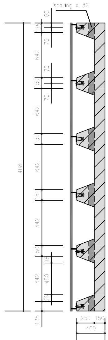
Langsdoorsnede
