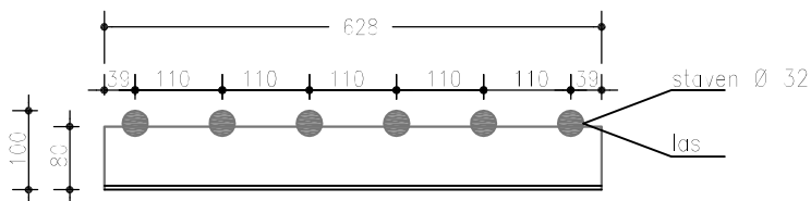
Aanzicht L 80.80.10
