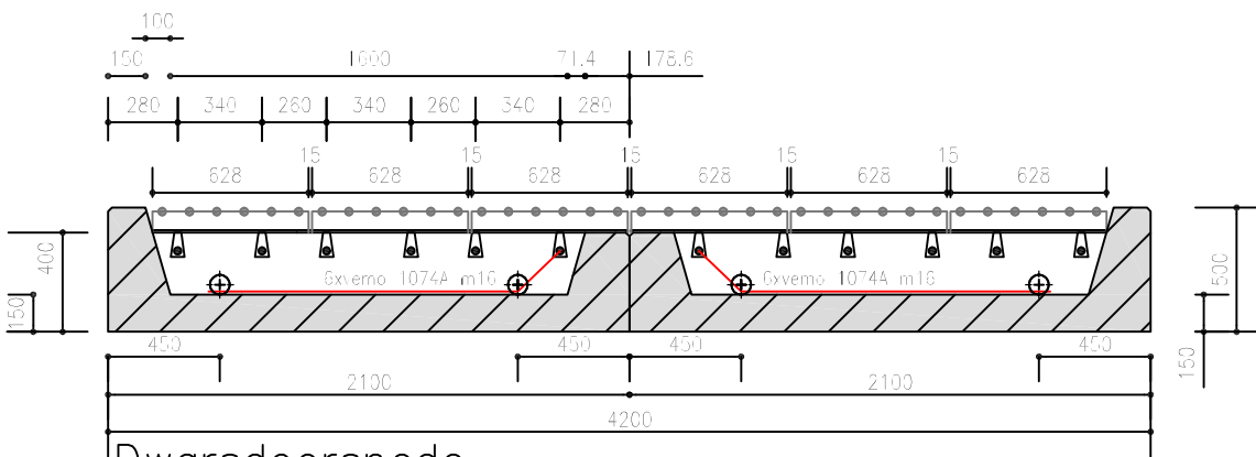
Dwarsdoorsnede
