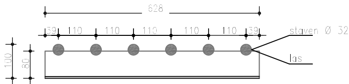
Aanzicht L 80.80.10
