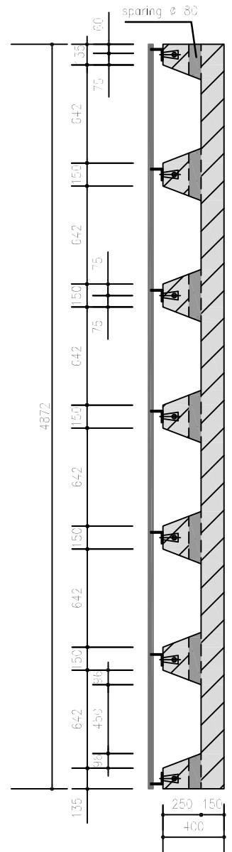
Langsdoorsnede
