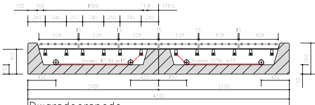
Dwarsdoorsnede
