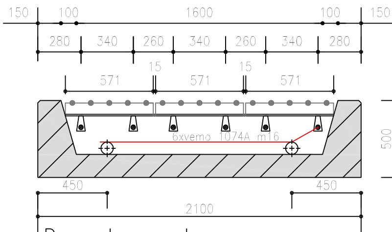
Dwarsdoorsnede
