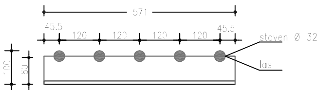
Aanzicht L 80.80.10
