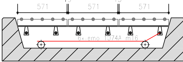
Dwarsdoorsnede
