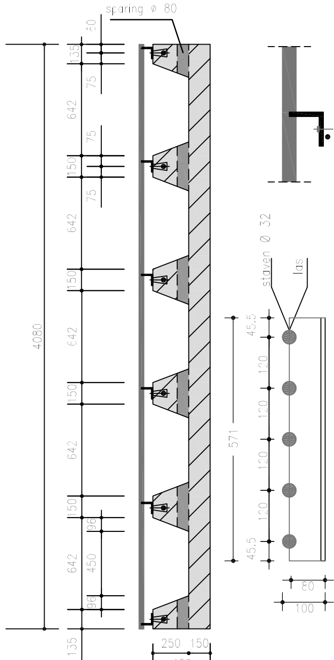
Langsdoorsnede
