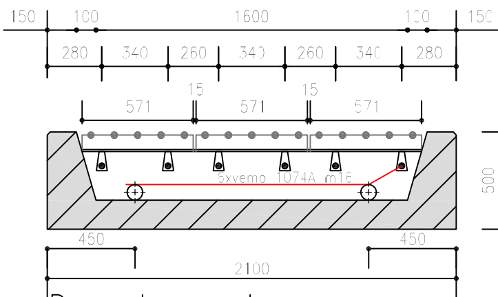
Dwarsdoorsnede
