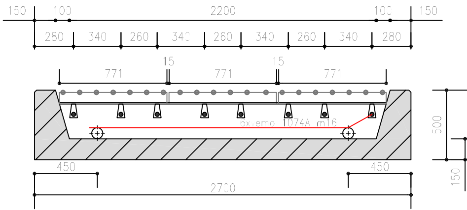
Dwarsdoorsnede
