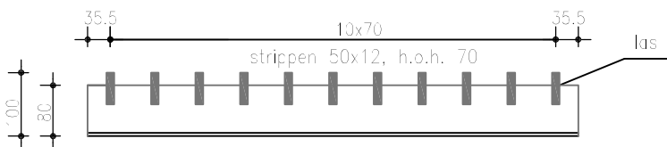
Aanzicht L 80.80.10
