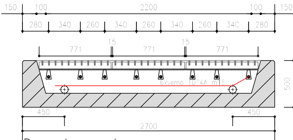
Dwarsdoorsnede
