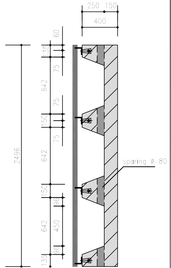
Langsdoorsnede
