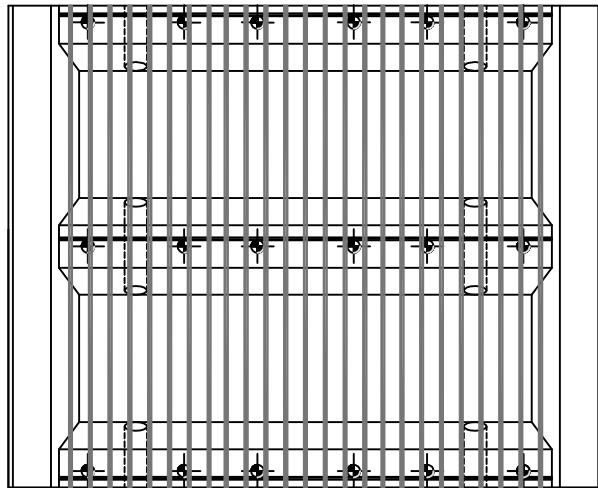
Bovenaanzicht
